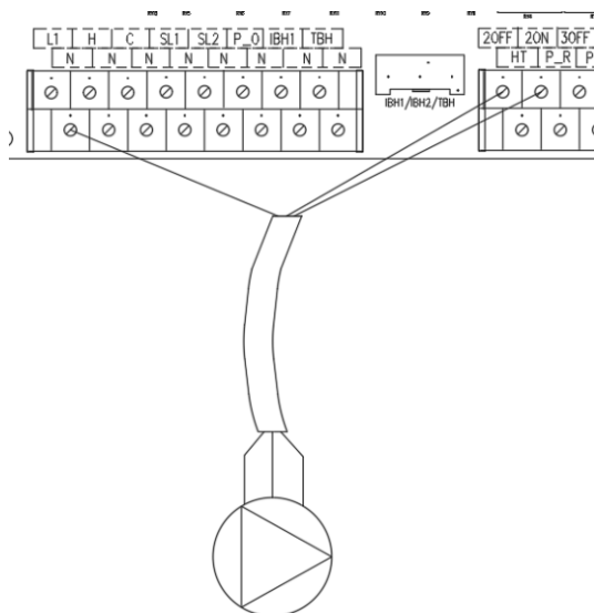
2# Электромагнитный 3-ходовой клапан
